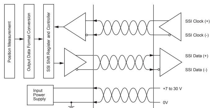
SSI Sensor Input
