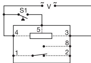
1. SPDT 8 Pin
